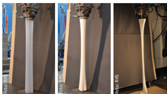
Abbildung 1: Vorformlingsbildung im Extrusionsversuch
