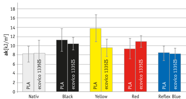
Abbildung 2: Schlagzähigkeitsergebnisse nach 14-tägiger UV-Bestrahlung
