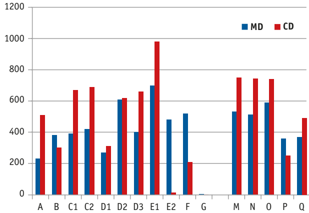
Abbildung 3: Bruchdehnung [%]
