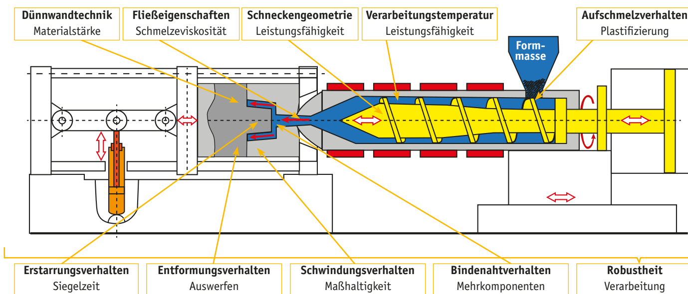
Abbildung 1: Faktoren mit Auswirkungen auf den Spritzgießprozess
